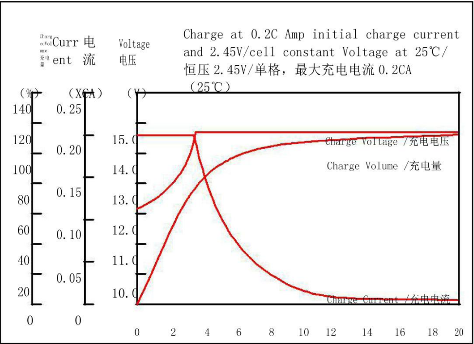
充电特性
