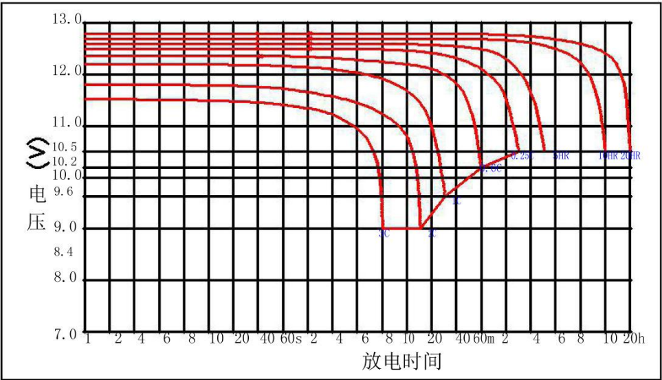
放电特性
